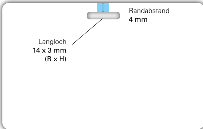
Platzierung Langloch
